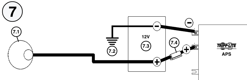
Basic 12VDC Vehicular Battery Connection. See Pg.8. 7.1 is the alternator. 7.2 is the vehicle battery ground. 7.3 is the vehicle battery. 7.4 is the fuse. Conexión Básica de Baterías de 12V de CD en Vehículos. Vea página 24. 7.1 representa el alternador. 7.2 representa la conexión a tierra de la batería del vehículo. 7.3 representa la batería del vehículo. 7.4 representa el fusible.
